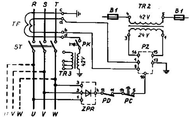
Rys. nr 4 Układ połączeń obwodu ziemnozwarciowego / odmiana 23 /
