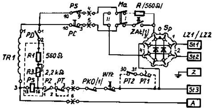
Rys. nr 2 Obwód sterowania wyłącznika
