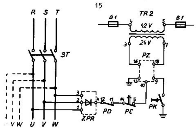
Rys. nr 3 Układ połączeń obwodu ziemnozwarciowego / odmiana 24 /
